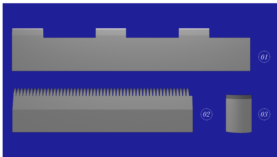
N°1 Couteau de prédécoupe transversale N°2 Couteau de prédécoupe longitudinale N°3 Onglet coupe blister
