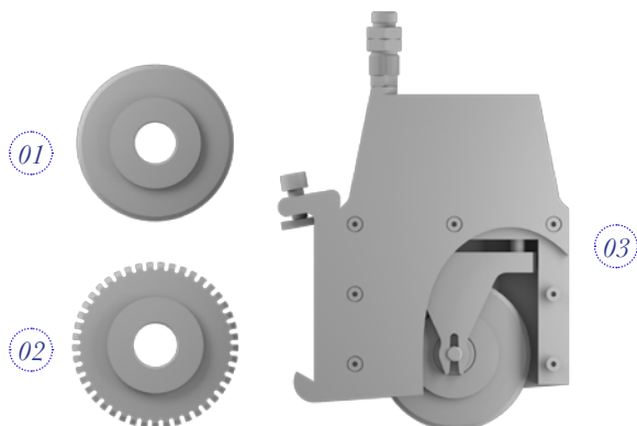
1 / Molette lisse 2 / Molette de perforation 3 / Ensemble molette/porte couteau pneumatique
